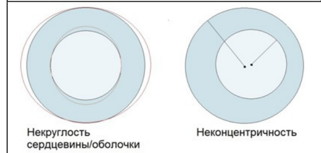
Рис. 3. Некруглость и неконцентричность сердцевинки и оболочки
