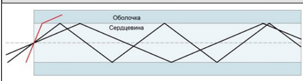
Рис. 2. Полное внутреннее отражение в оптическом волокне
