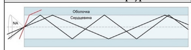
Рис. 4. Числовая апертура
