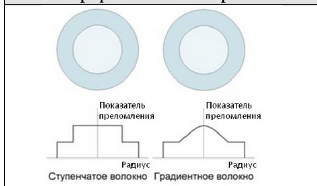
Рис. 5. Профили показателя преломления
